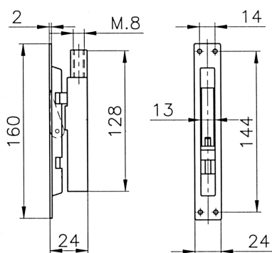
EB 198 – egyirányú megerősített fémajtó tolózár
