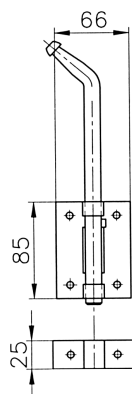
BC 318 / 250 tolózár rajza.
