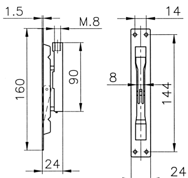
EB 194 – egyirányú fémajtó tolózár
