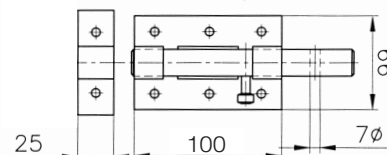
ZIUR 454 / 100-as méretű tolózár rajza.
