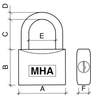
Hagyományos kengyelű lakat
