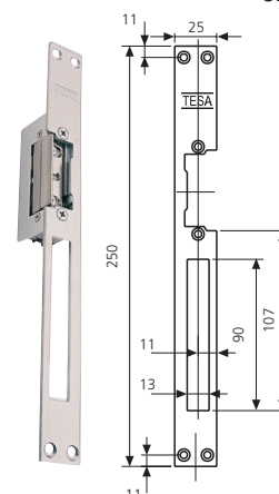
LCI Hagományos zárnyelvű zárhoz
