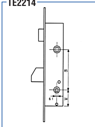
WC ráfordítós zár
