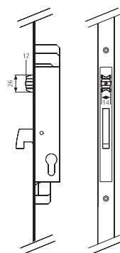
Lengőajtó zár
