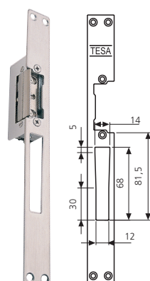
LBI Kicsapódó, ferde nyelvű zárhoz
