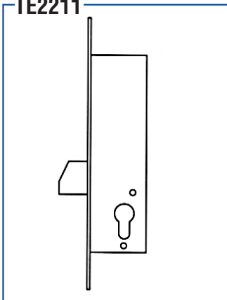
Bejárati ajtó kilincsnyelv nélkül
