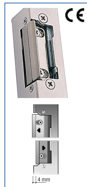
A kilincsnyelv fogadó oldalirányú állíthatósága
