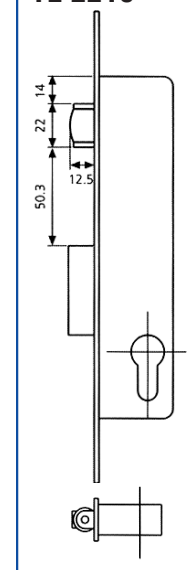
Lengőajtó zár
