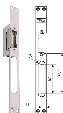
BUI Hengeres zárnyelvű zárhoz
