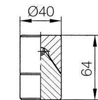
Alsó forgótengely
