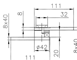
Felső forgótengely
