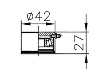
Alsó forgótengely
