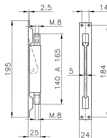
EB 199 – kétirányú fémajtó tolózár
