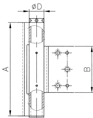
Tűzálló pánt rugó nélkül
