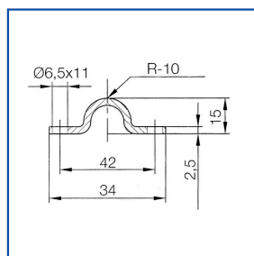
Gömbölyű sín Ebro 535 / 3 m
