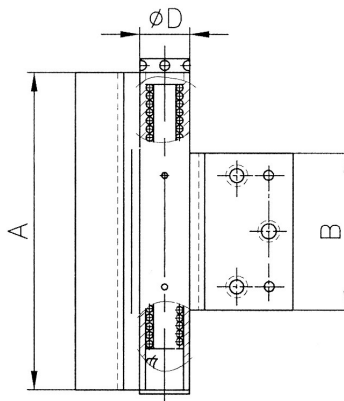
Tűzálló pánt rugóval
