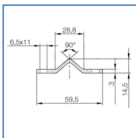
Derékszögű V sín Ebro 537 / 3 m
