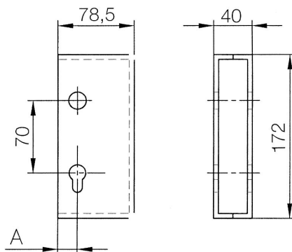
Ebro kampós zár megerősített zárháza
