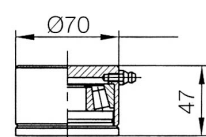
Alsó forgótengely
