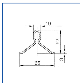
10-as sín Ebro 536 / 3 m
