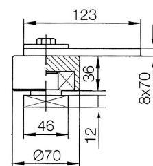
Felső forgótengely
