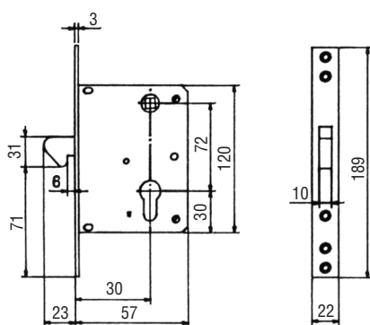
Ebro 4240 kampós zár
