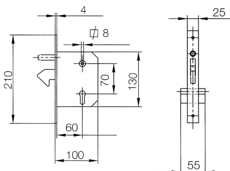
Ebro 3250 kampós zár
